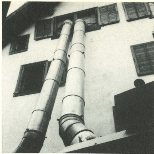
Eine spektakuläre Phase gleich zu Beginn der Umbauarbeiten: das gesamte Holzwerk wird mit Heissluft gegen Schädlinge geschützt. Durch grosse Rohre wird über 70 °C heisse Luft während Stunden in die völlig abgedichteten Räume geblasen.
